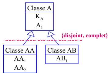
Diagramme de classes
