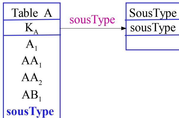
modèle relationnel
