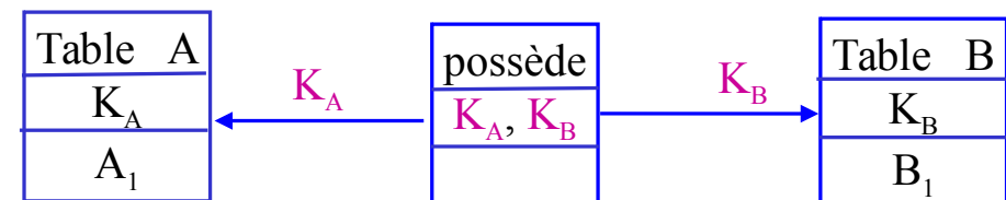
modèle relationnel
