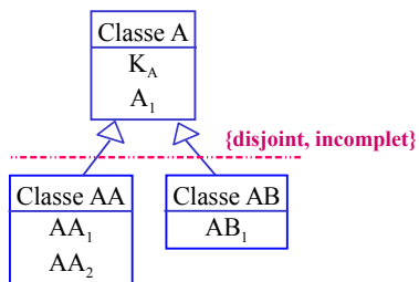
Diagramme de classes
