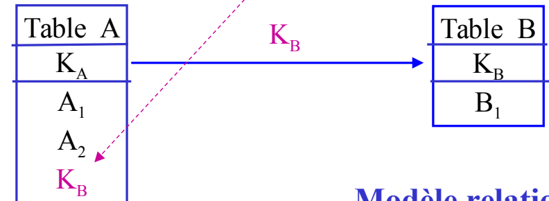
Modèle relationnel
