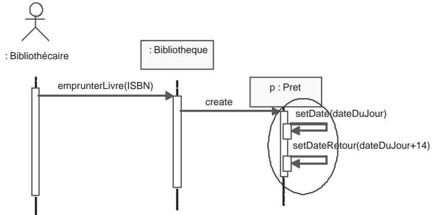
Figure 8-9. Diagramme de séquence de l'opération emprunterLivres (suite 2)
