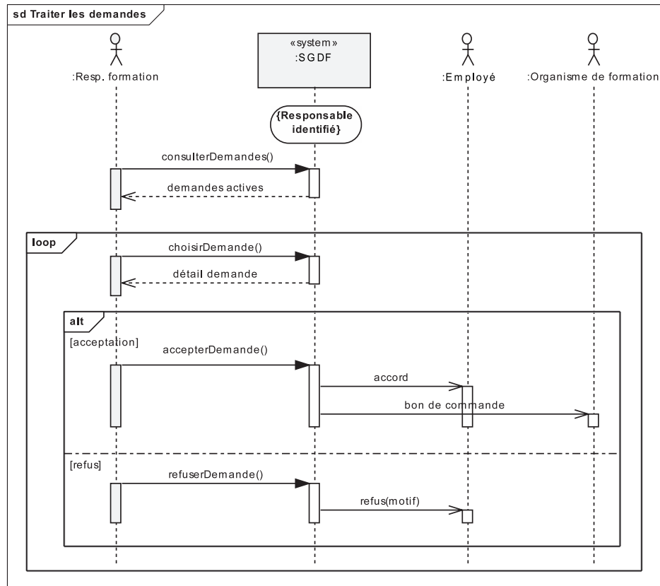
Figure 7-64. Diagramme de séquence système de Traiter les demandes
