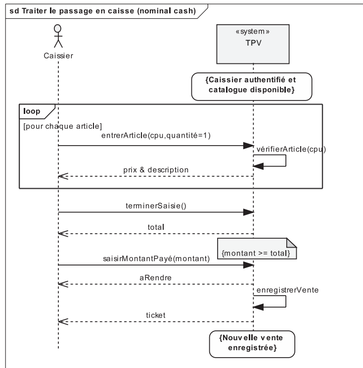
Figure 2-7. Version plus élaborée du DSS du scénario nominal de Traiter le passage en caisse
